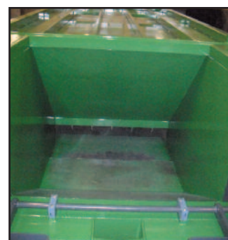
Auget grande dimension, sans aspérité pour éviter la rétention des déchets (Big burnished Loading bay to avoid waste retention)
