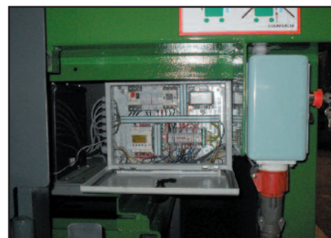
• Coffret électrique protégé dans le local technique (Protected Electric Panel inside the technical premise)
